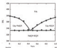
電解質 NaFSa-KFSA 二元系状態図
