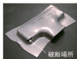
実測限界ストローク = 17.8 mm 実験結果
