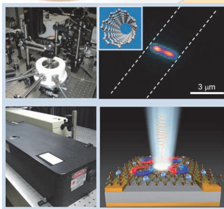
先端レーザー分光システムと 極限ナノ物質の光学イメージ等
