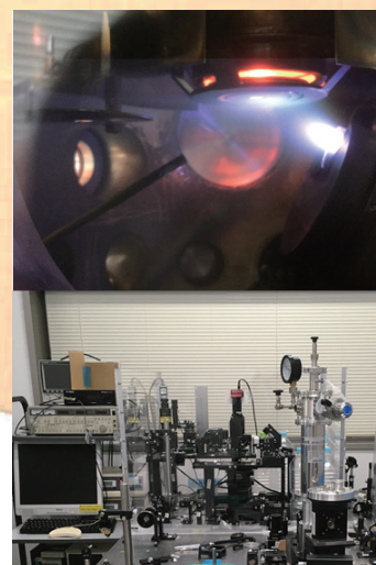
パルスレーザー蒸着による成膜の様子（上）と テラヘルツ分光・イメージングシステム（下）
