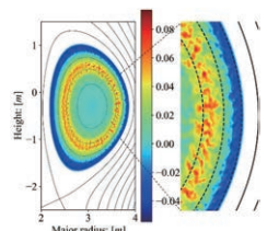
核融合炉を想定した非円形 断面プラズマ中の乱流
