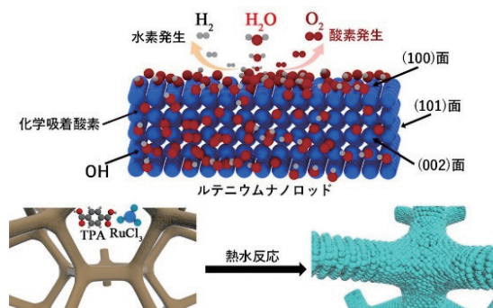
高活性触媒による水の電気分解
