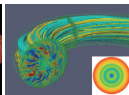
核融合プラズマ中の乱流。 自己組織的に形成された 環状流を伴う（右下）
