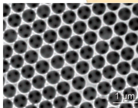
ZnO 三次元フォトニック結晶
