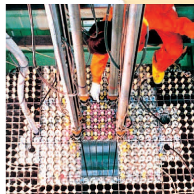
臨界集合体を用いた実験風景
