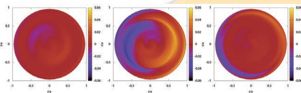
ビーム放射分光法によって計測した プラズマ断面の密度揺らぎの時間発展 不安定性が発生するたびに形成・消失する 揺らぎのらせん構造を非線形解析で解明
