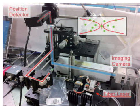
レーザートラップ装置
