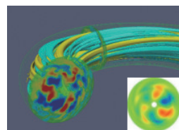
磁場構造形成を伴う（右下） 核融合プラズマ中の乱流
