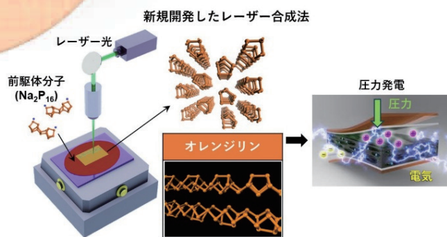
発電する新規リン同素体 (オレンジン)
