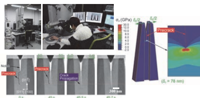
透視型電子顕微鏡内の破壊実験の様子と 応力解析結果
