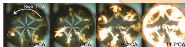
ボトムビュー可視化エンジンによる火炎挙動の解析
