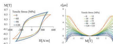
電磁気材料のマルチフィジックス解析
