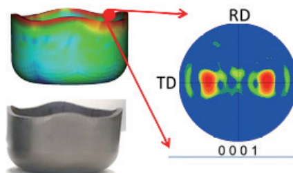
純チタン板の円筒絞り成形に関する実験と マルチスケール結晶塑性シミュレーション
